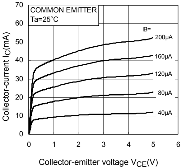
I_C-V_{CE}
