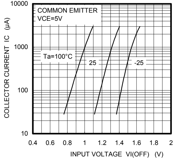
IC - VI(OFF)
