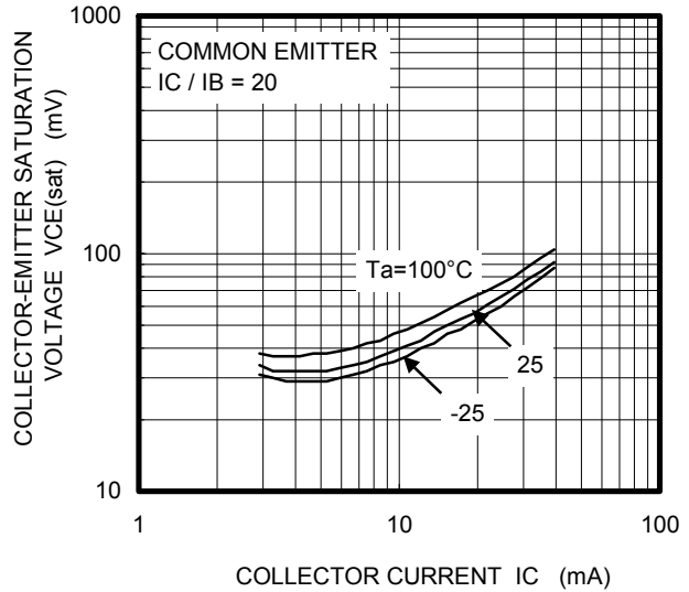
VCE(sat) - IC
