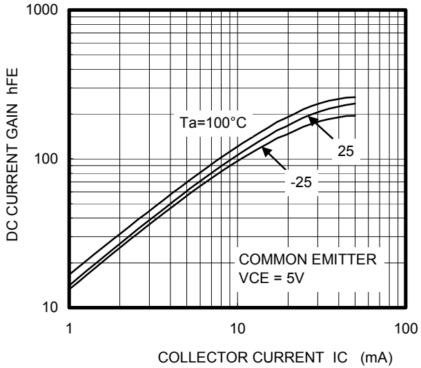
hFE - IC
