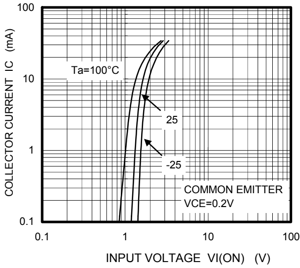
IC - VI(ON)
