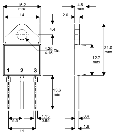
SOT93
