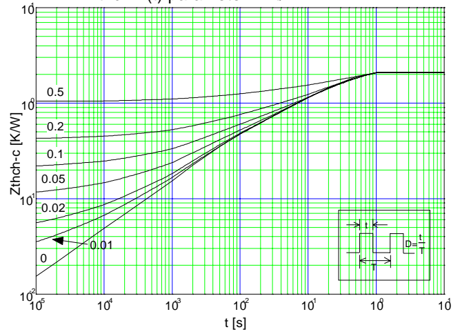
Transient thermal impedance Z_{thch}=f(t) parameter: D=t/T
