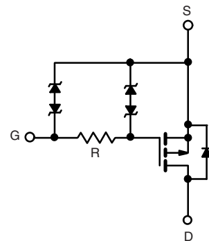
P-Channel MOSFET
