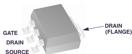
SOT-223
