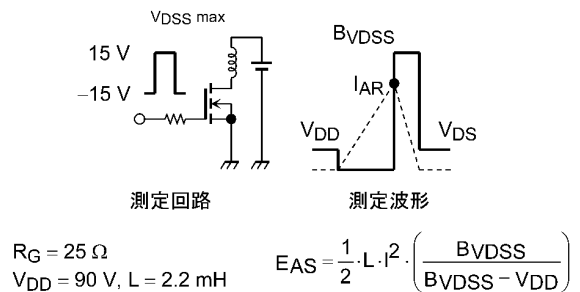
図 8.16 測定回路/測定波形
