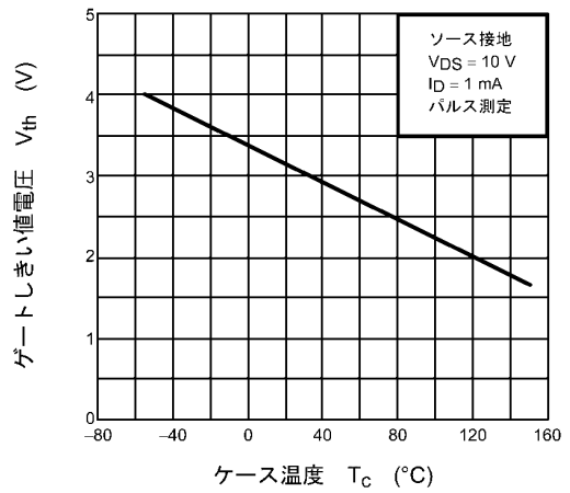
図 8.10 V_{th} - T_c
