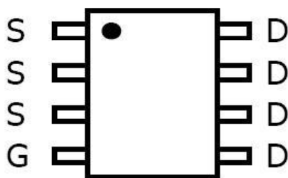
SOP-08
