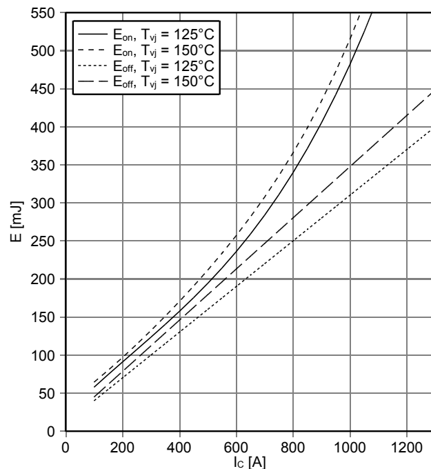
スイッチング損失 IGBT、チヨッパー (Typical) switching losses IGBT-Chopper (typical)
