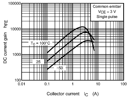
Fig. 7.4 h_{FE} - I_C
