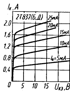
Выходные характеристики
