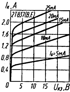
Выходные характеристики
