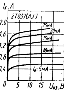
Выходные характеристики
