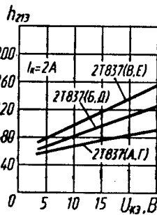
Зависимость статического коэффициента передачи тока от напряжения коллектор—эмиттер
