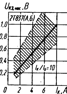
Зона возможных положений зависимости напряжения насыщения коллектор—эмиттер от тока коллектора
