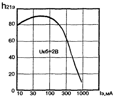
Зависимость статического коэффициента передачи тока от постоянного тока эмиттера
