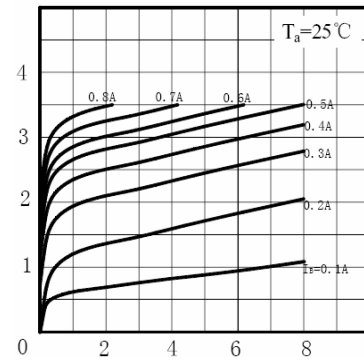
V_{BES}-I_c
