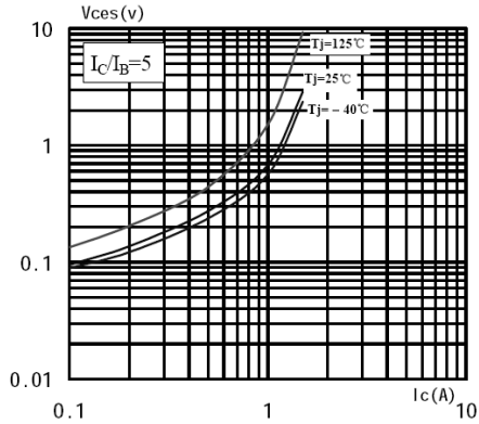
V_{ces} - I_c
