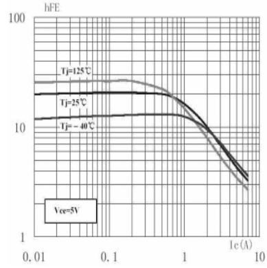
h_{FE} - I_C
