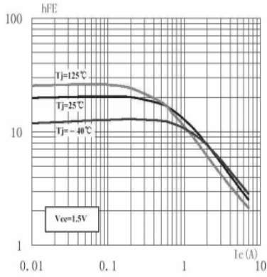
h_{FE} - I_C
