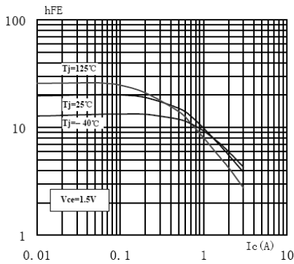
h_{FE} - I_c
