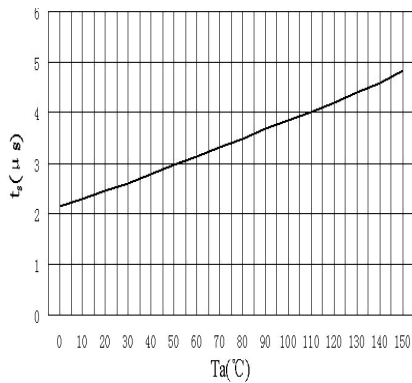
t_s - T_a
