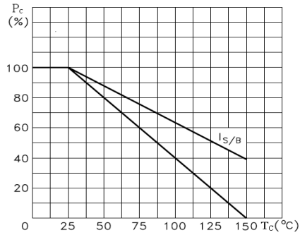
P_c - T_c
