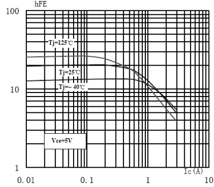
h_{FE} - I_c
