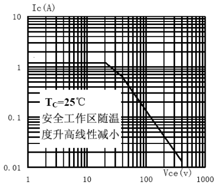
SOA (DC)
