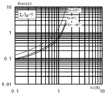
V_{ces} - I_C
