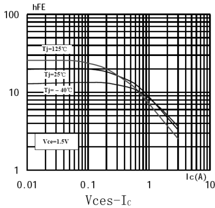
h_{FE} - I_C
