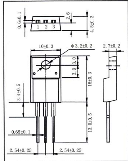
T0-220F 单位: mm
