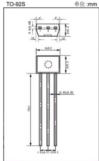
引脚：1.S 2.G 3.D
