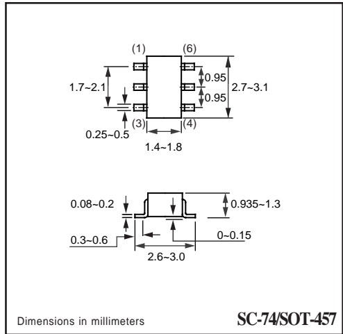
SC-74/SOT-457
