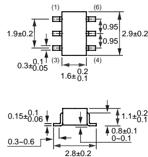
SC-74/SOT-457
