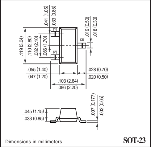
SOT-23
